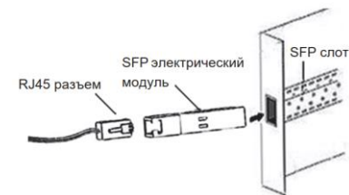
Рис. 2. Подключение электрического модуля SFP
